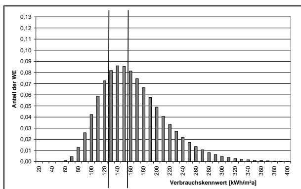
Abb. 41: Verteilung Gas ABL normiert
