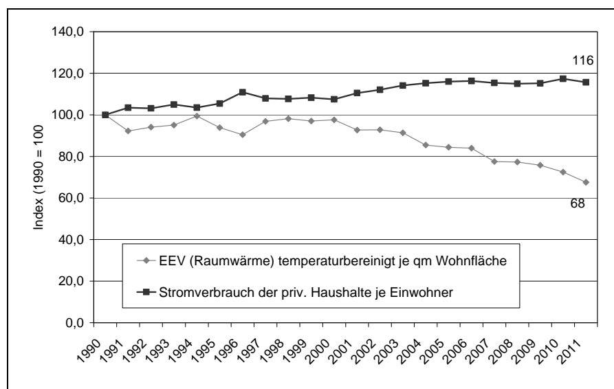
Abb. 58: Entwicklung des Endenergieverbrauchs (EEV) für Raumwärme pro m 2 Wohnfläche und des Stromverbrauchs privater Haushalte je Einwohner seit 1990, [BMWi 2013], eigene Darstellung
