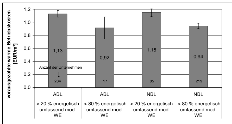
Abb. 35: Mittlere vorausgezählte warme Betriebskosten 2010 mit Angabe des Vertrauensbereiches, Konfidenzintervall 0,95
