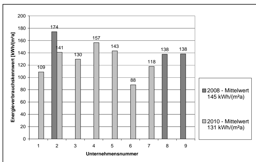
Abb. 42: Mittlere Energieverbrauchskennwerte für Gebäude mit Gasetagenheizung in Berliner Wohnungsunternehmen, gradtagsbereinigt. Datengrundlage 2008: 3 Unternehmen, 270.000 m 2 mit GEH, 2010: 7 Unternehmen, 300.000 m 2 mit GEH,
