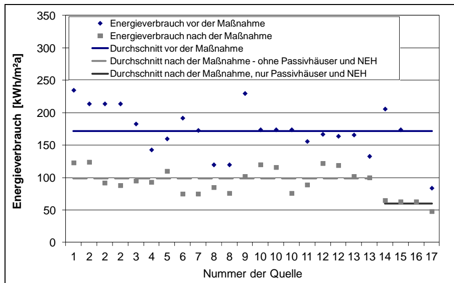
Abb. 43: Energieverbrauch vor und nach energetischer Modernisierung entsprechend der in Tabelle 18 analysierten Quellen
