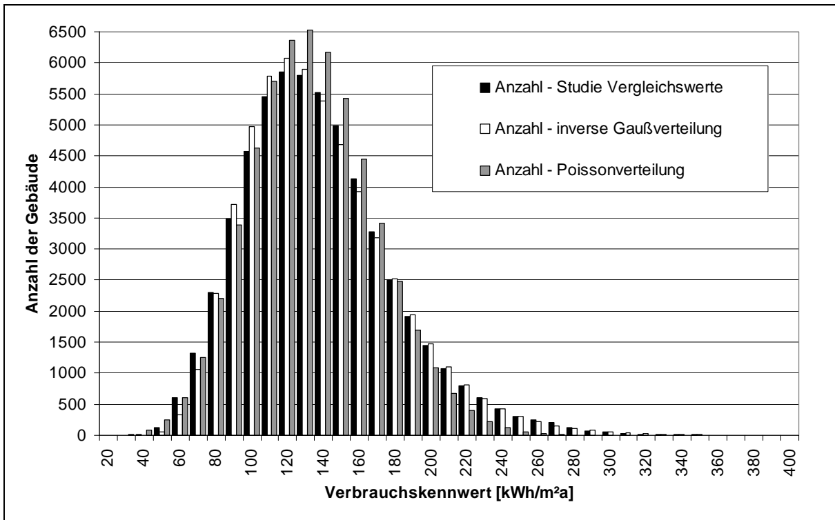
Abb. 119: Verteilung aus Abb. 115, ergänzt um inverse Gaußverteilung und Poissonverteilung jeweils angepasst mit den geringsten Abweichungsquadraten (best fit)
