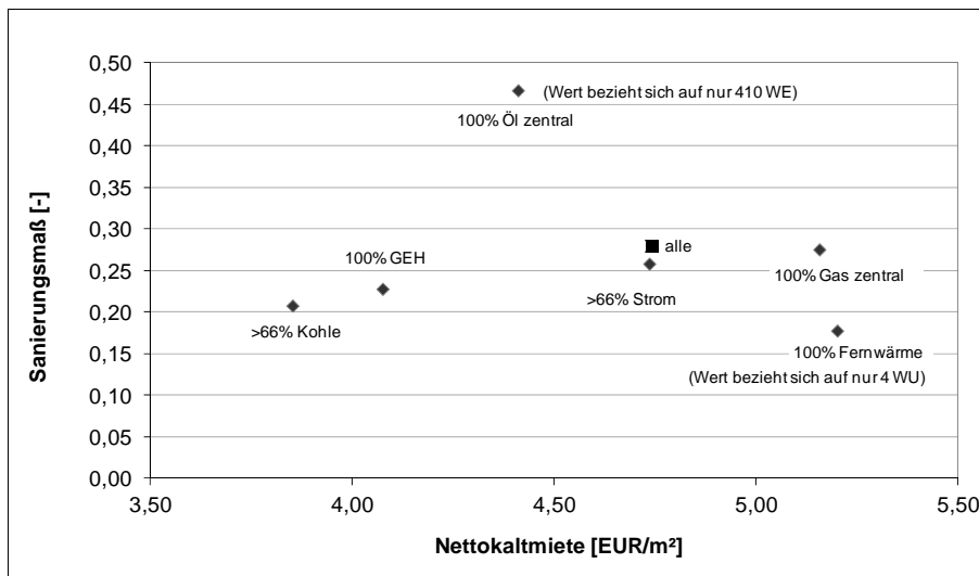
Abb. 27: Zusammenhang zwischen Nettokaltmiete und Sanierungsmaß für verschiedene Beheizungsformen, ABL
