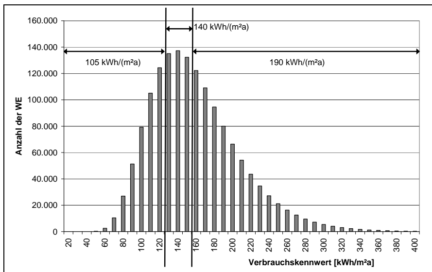
Abb. 39: Verteilung der Energieverbrauchskennwerte für gaskesselversorgte Objekte, ca. 1,5 Mio. WE bei den Wohnungsunternehmen, einschließlich mittlerer Energieverbrauchskennwerte für seit 1990 neuerrichtete oder umfassend energetisch modernisierte / energetisch teilmodernisierte / energetisch unmodernisierte Objekte, inverse Gaußverteilung, Mittelwert 159 kWh/(m 2 ), Schiefe 0,93
