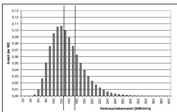
Abb. 40: Verteilung Gas NBL normiert
