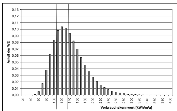
Abb. 38: Verteilung FW ABL normiert
